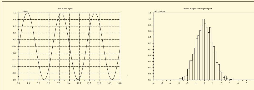
圖 6.13: Blatexp2 Example
